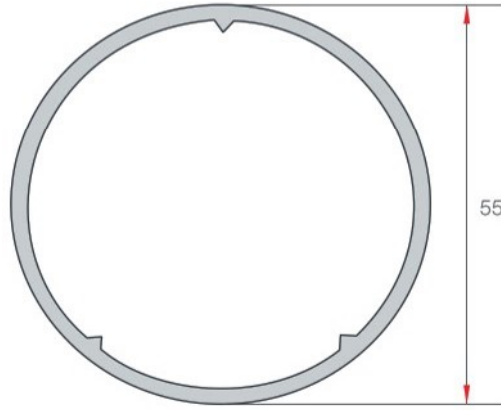
Ø 50 BORU PIPE PROFILE EN 58
