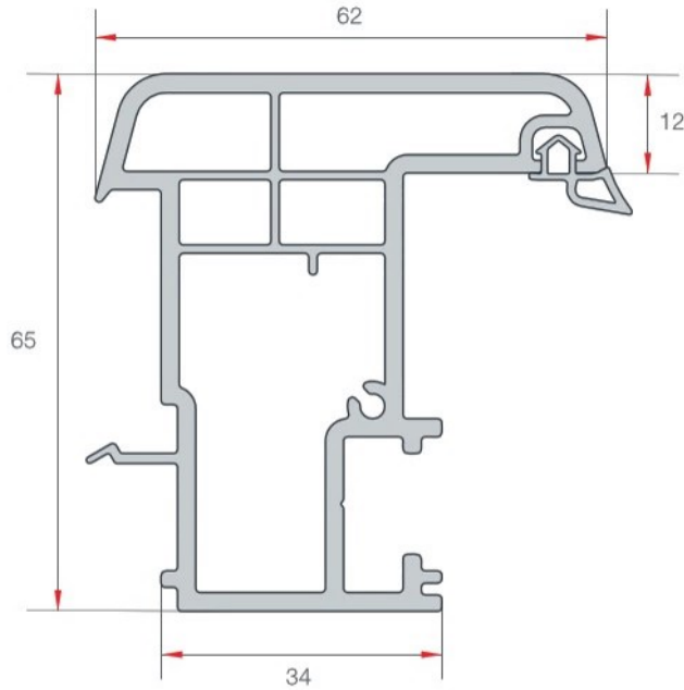
KLASLINE HAREKETLİ ORTA KAYIT PROFİLİ KLASLINE MOVABLE MULLION PROFILE EN 24
