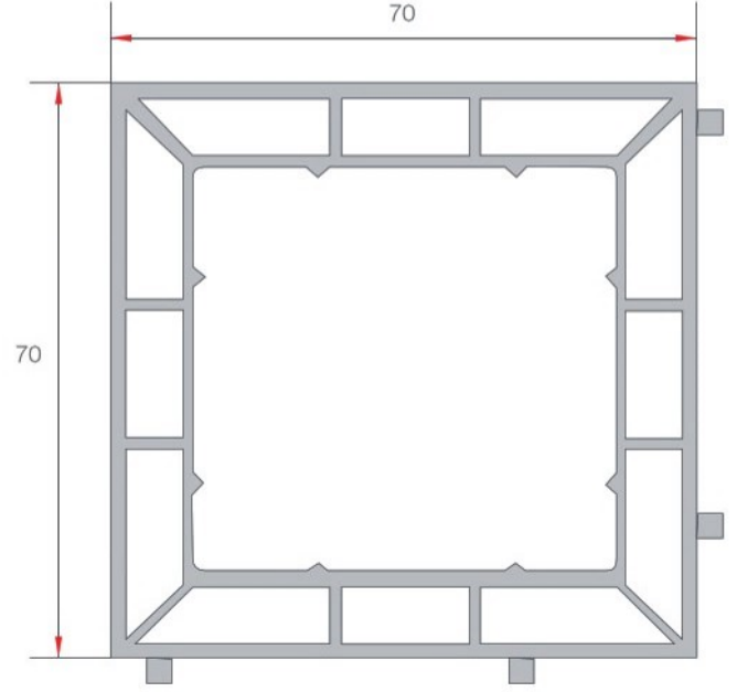
70 x 70 KUTU 70 x 70 BOX PROFILE EN 55
