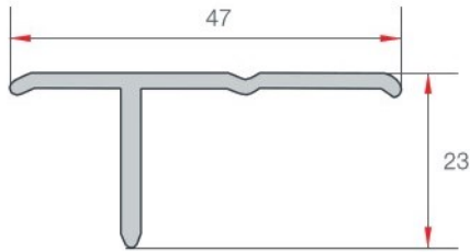
ASİMETRİK "T" PROFİLİ ASYMETRIC "T" PROFILE EN 64
