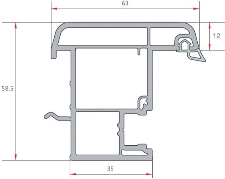
VIZYONLINE HAREKETLİ ORTA KAYIT VIZYONLINE MOVABLE MULLION PROFILE EN 25
